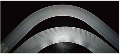
帯板の面内曲げ
