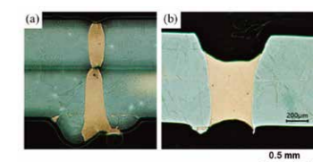
軟磁性材に浸入させたCu融体
