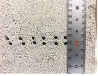
削孔試験後の削孔跡
