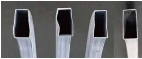
極薄肉方形管の回転引曲げによる断面変形
