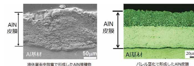
Al表面へのAlNの形成
