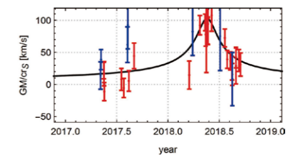
一般相対論効果の検出結果
