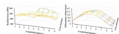
残留応力と材料変形のマッピング
