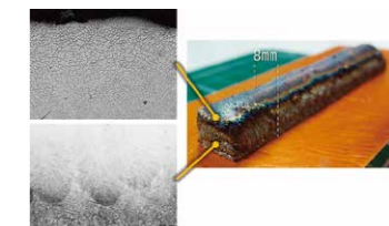
SKD61積層造形材と金属組織
