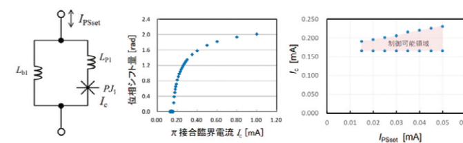
新奇超伝導回路の数値計算評価
