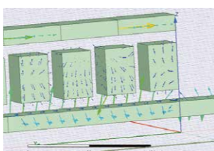
磁気シミュレーション
