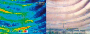
コンクリート製仏像の赤外線調査
