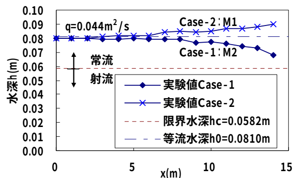
図-1.4 水面形 (Case-1, Case-2 の例) (上記は M1, M2 カーブの例)
