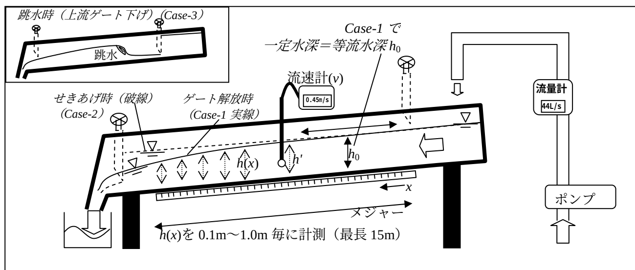
図-1.2 実験装置の概要
