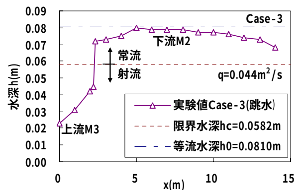
図-1.5 水面形 (Case-3 の例)
